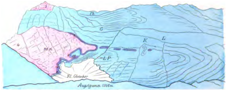
Fig. 1. Entlüftung des Hauptgneisskeils 4 am Gstellhorn, oberhalb der Alp Augtgamm. Ch Chorochsee, G - altes Gletscherbett, K - Kanzel, L - Leitern, LP - Leiternplatten.
